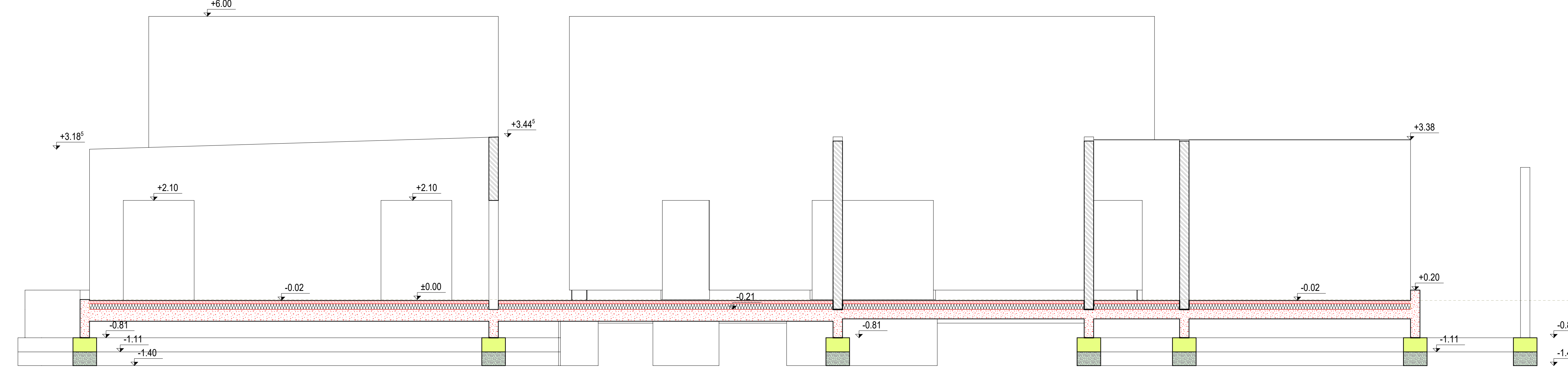
Coupe 5 - 5
