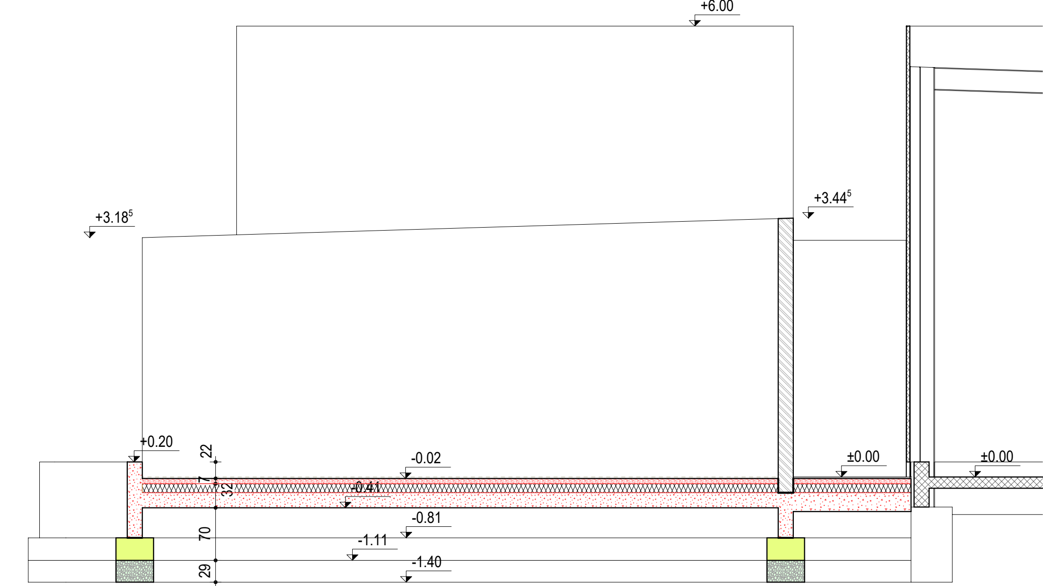
Coupe 4 - 4
