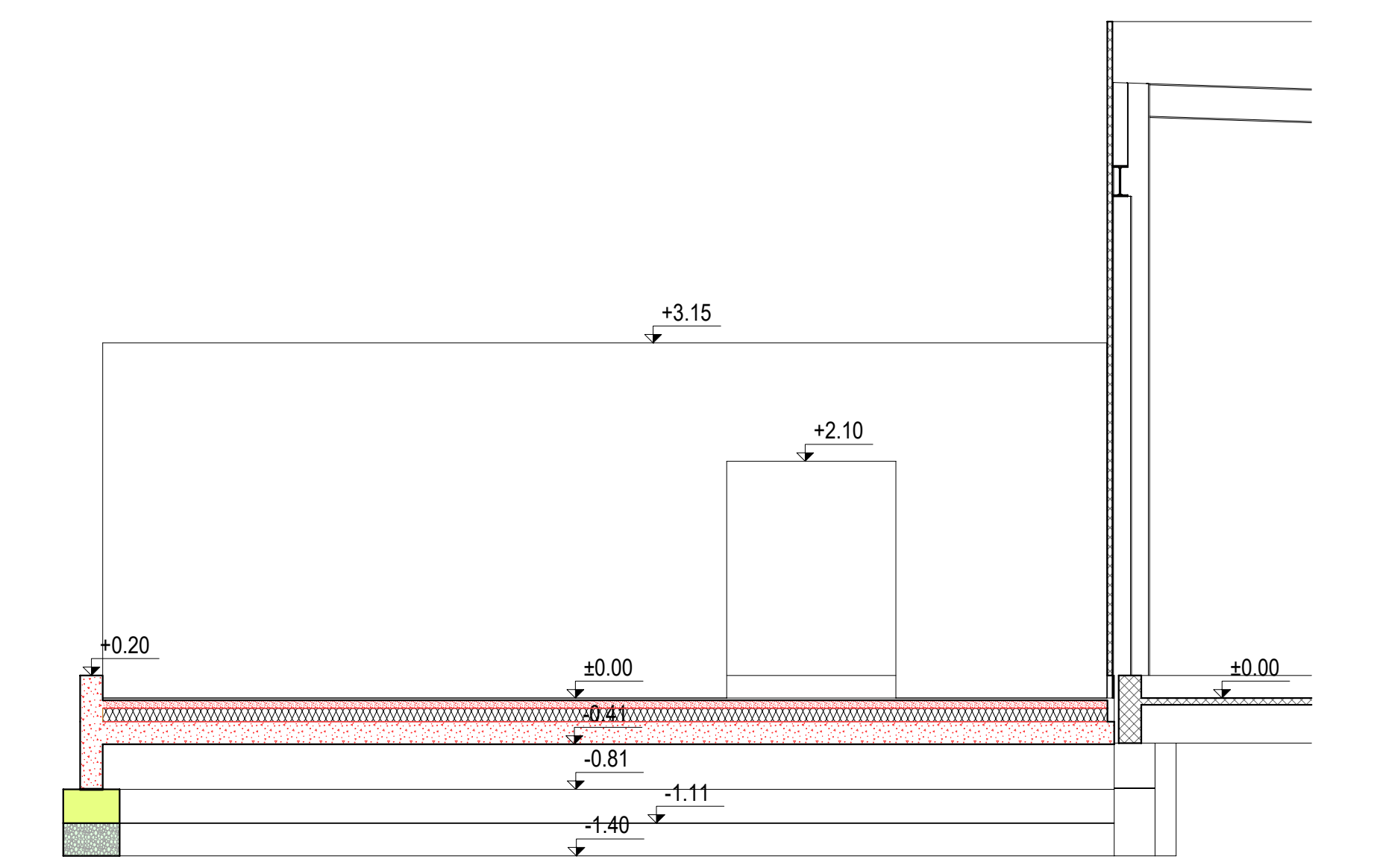
Coupe 3 - 3
