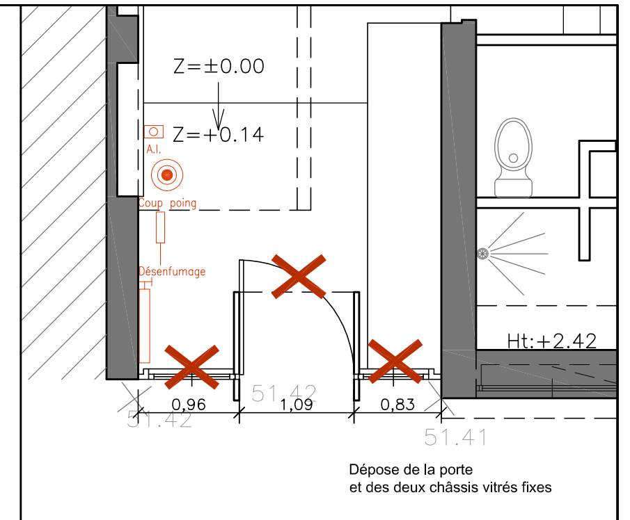
ZOOM SUR PORTE D'ACCES DU PERSONNEL TECHNIQUE - ETAT EXISTANT
