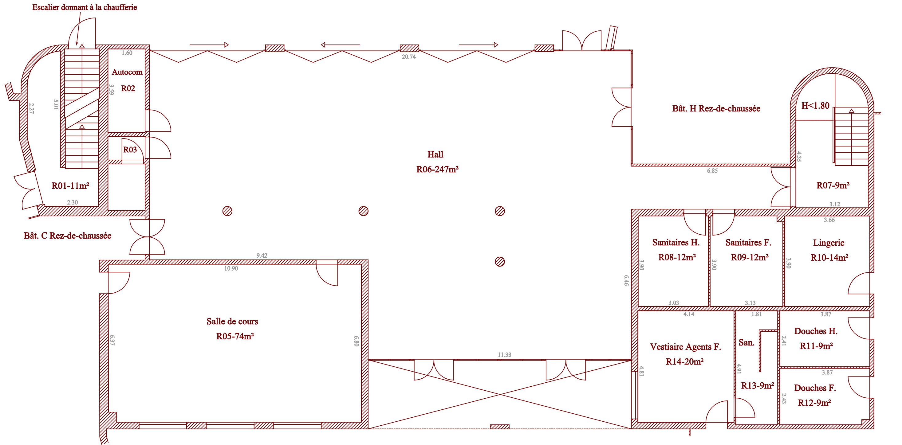
Bât. H Rez-de-chaussée
