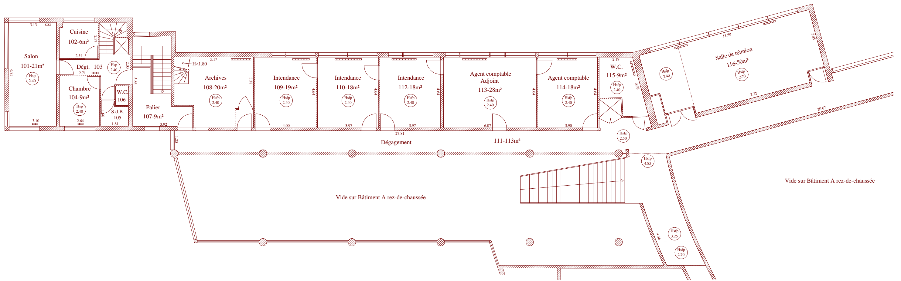
Bât. B étage 1
