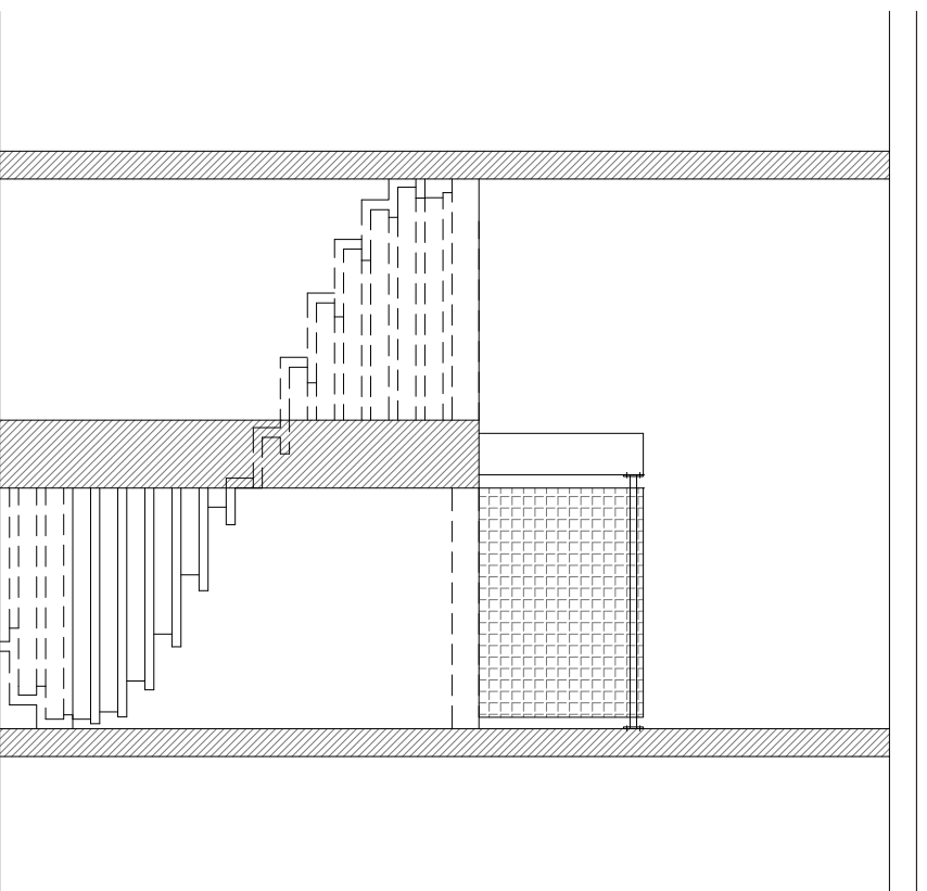
Coupe AA'
